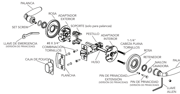
Despiece (Se muestra la función de privacidad)
