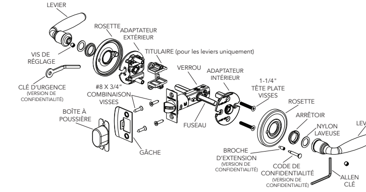
Vue éclatée (Fonction de confidentialité illustrée)
